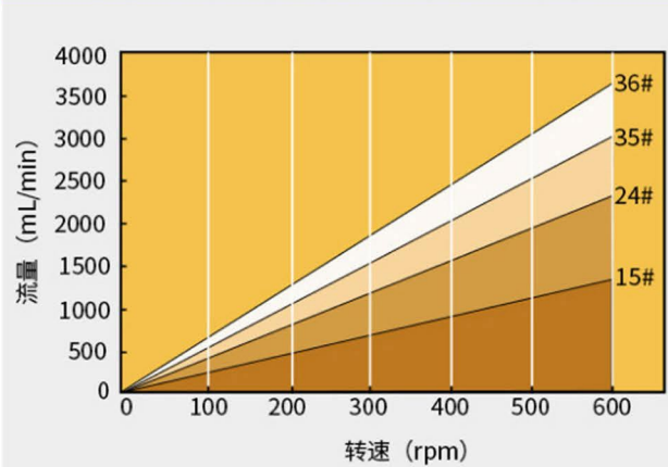
DZ25-3L泵头流量范围 (0.1-600rpm)
