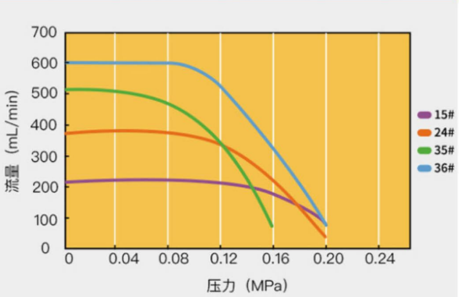
DZ25-3L泵头压力/流量曲线图 (100rpm)
